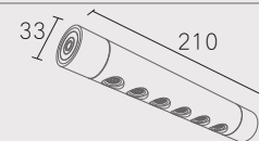
六头射灯拼接件
