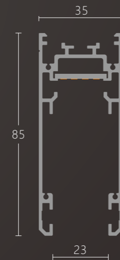
轨道截面尺寸图 (单位: mm)
