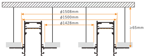
龙骨预埋式
