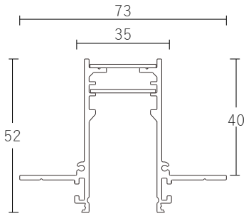
轨道截面尺寸图（单位：mm）
