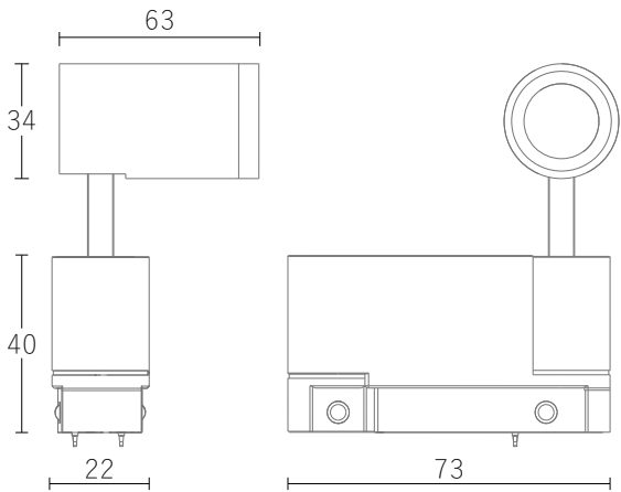
尺寸图 (mm)
