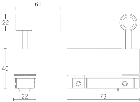
尺寸图 (mm)
