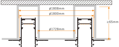
木盒预埋式
