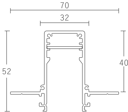
轨道截面尺寸图（单位：mm）
