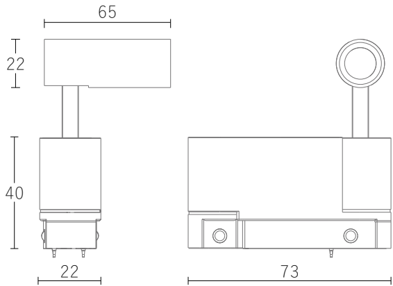
尺寸图 (mm)
