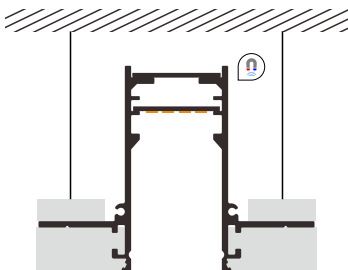
龙骨预埋式
