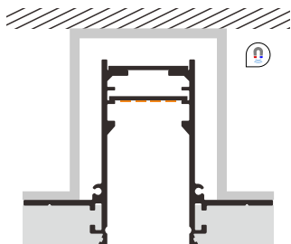
木盒预埋式
