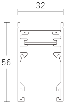
轨道截面尺寸图（单位：mm）
