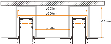
木盒预埋式
