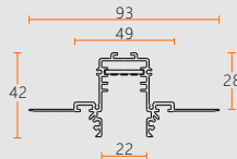
轨道截面尺寸图 (单位：mm)
