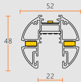
轨道截面尺寸图 (单位: mm)
