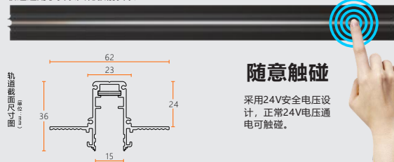
轨道适用于安装天花板前安装
