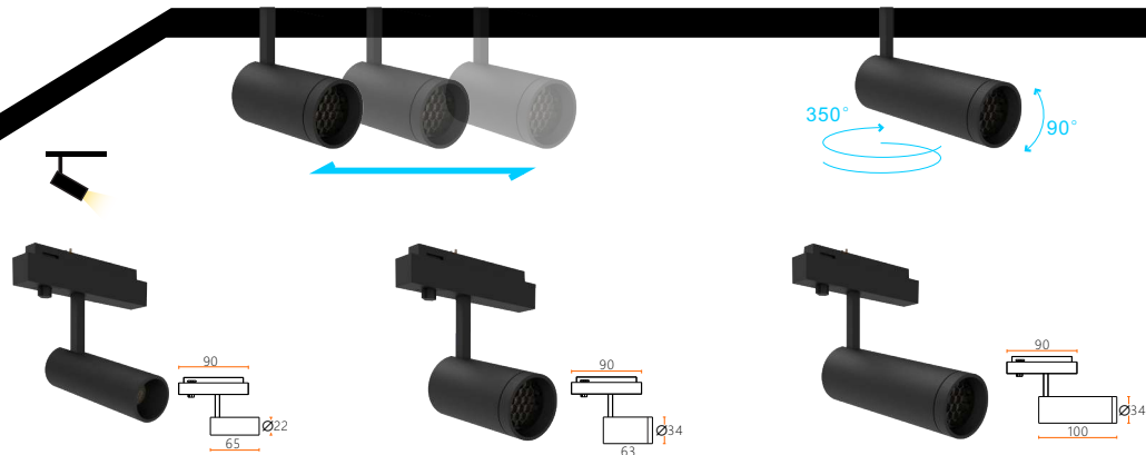
安装灯具后 旋转按钮锁定灯具
